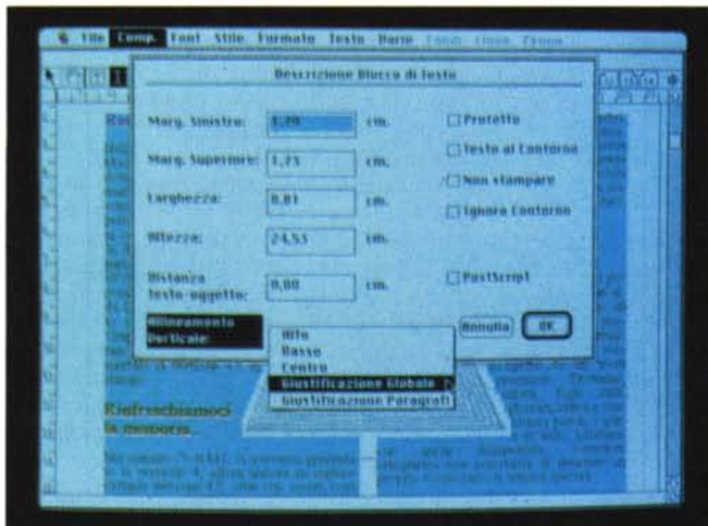
Foto 6 - La finestra che consente di indicare con precisione lo spostamento desiderato.
